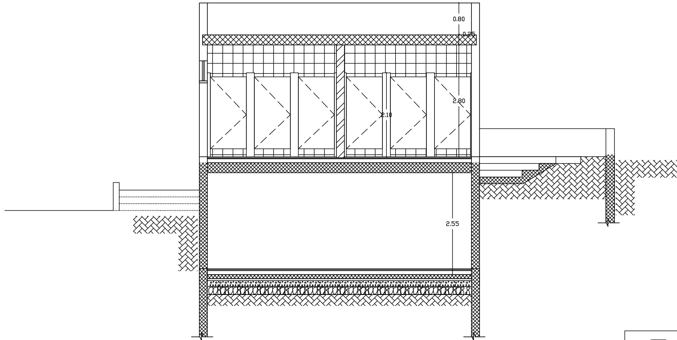
SECTION A-A
