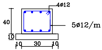
SEC. a-a
