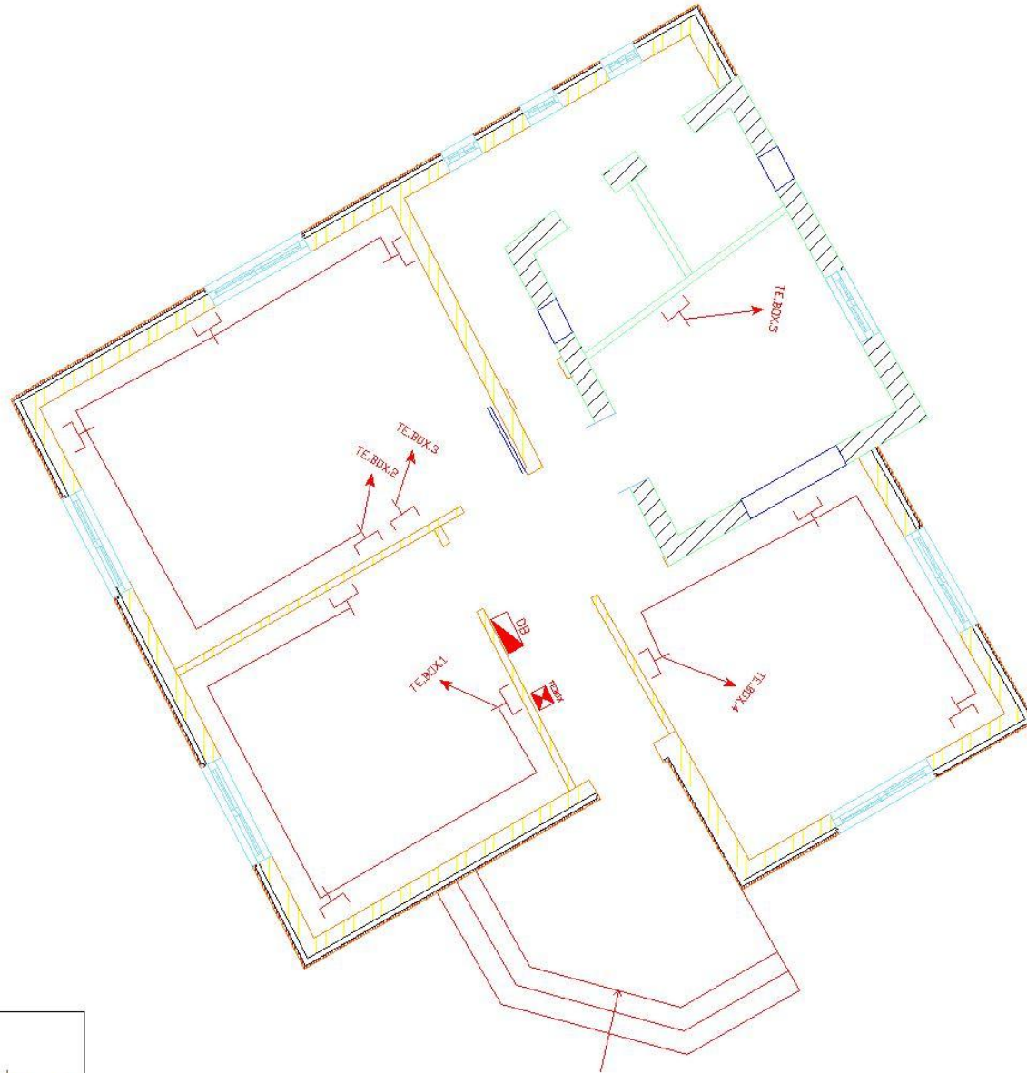
لوحة مخارج شبكة العوائف الداخلية
