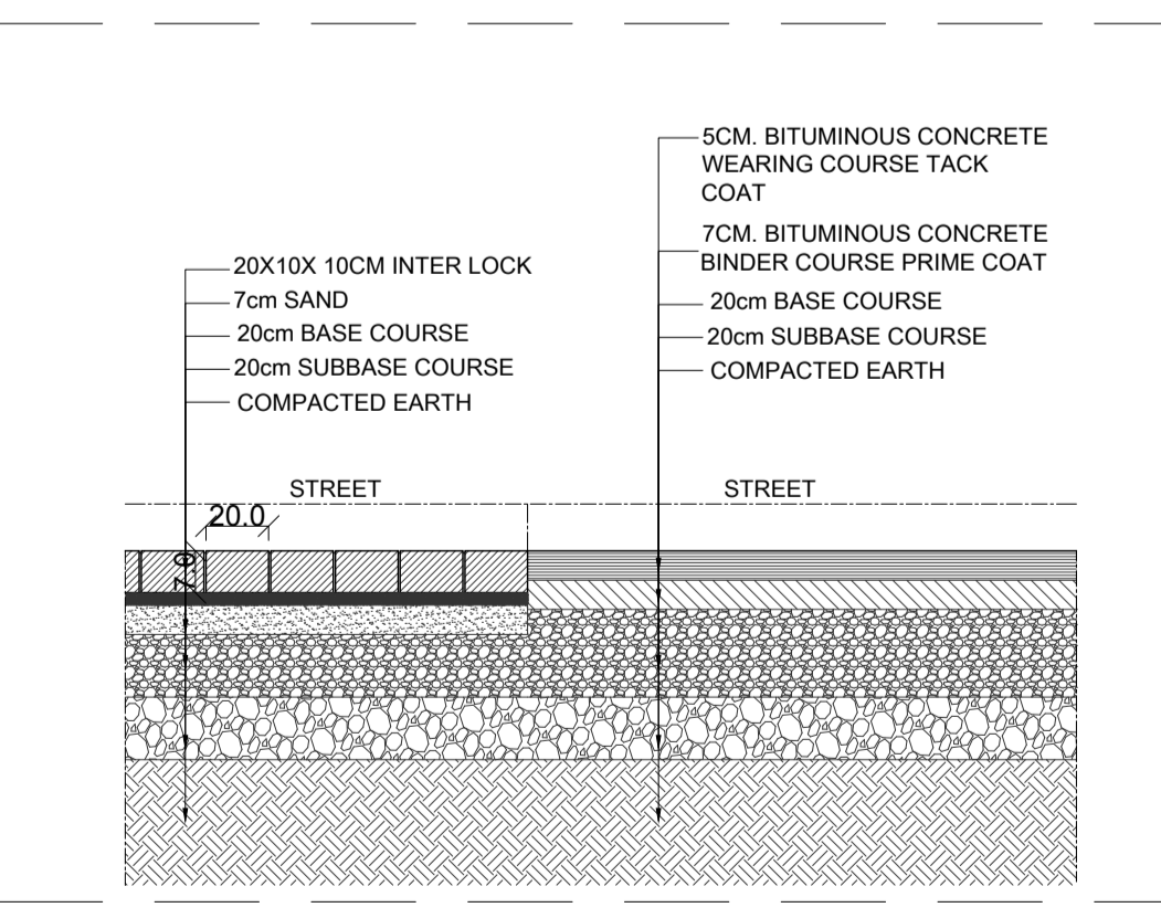
SECTION - S08 SCALE: 1-20
