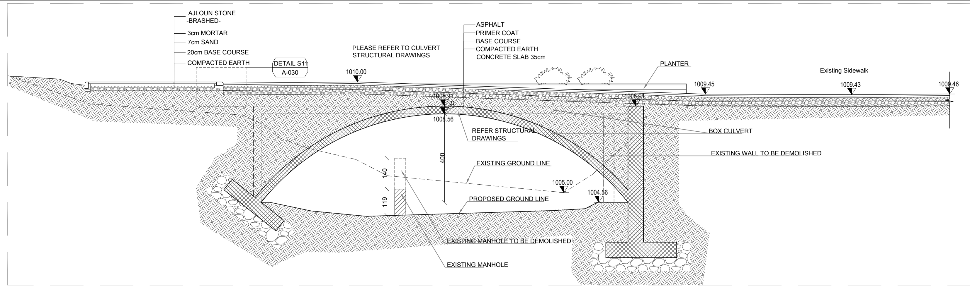
SECTION A-A
