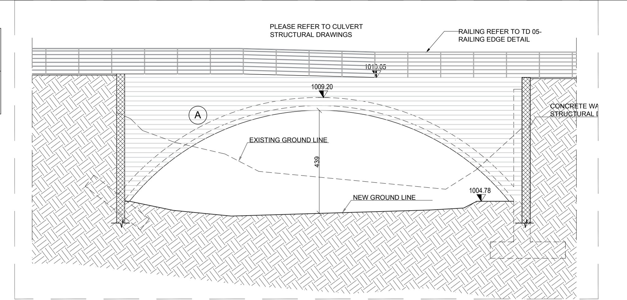
ELEVATION 01
