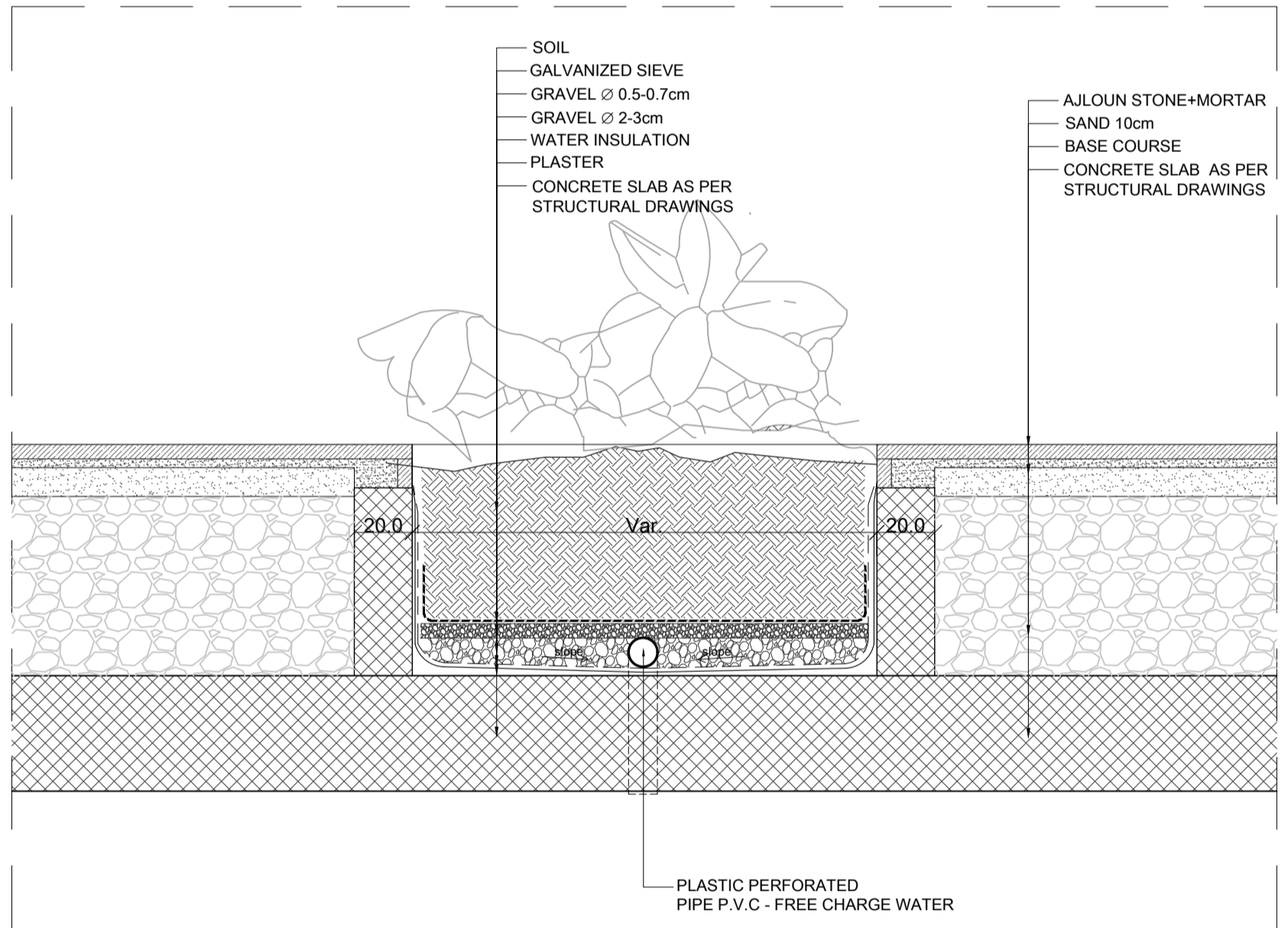
SECTION - S04 SCALE: 1-20
