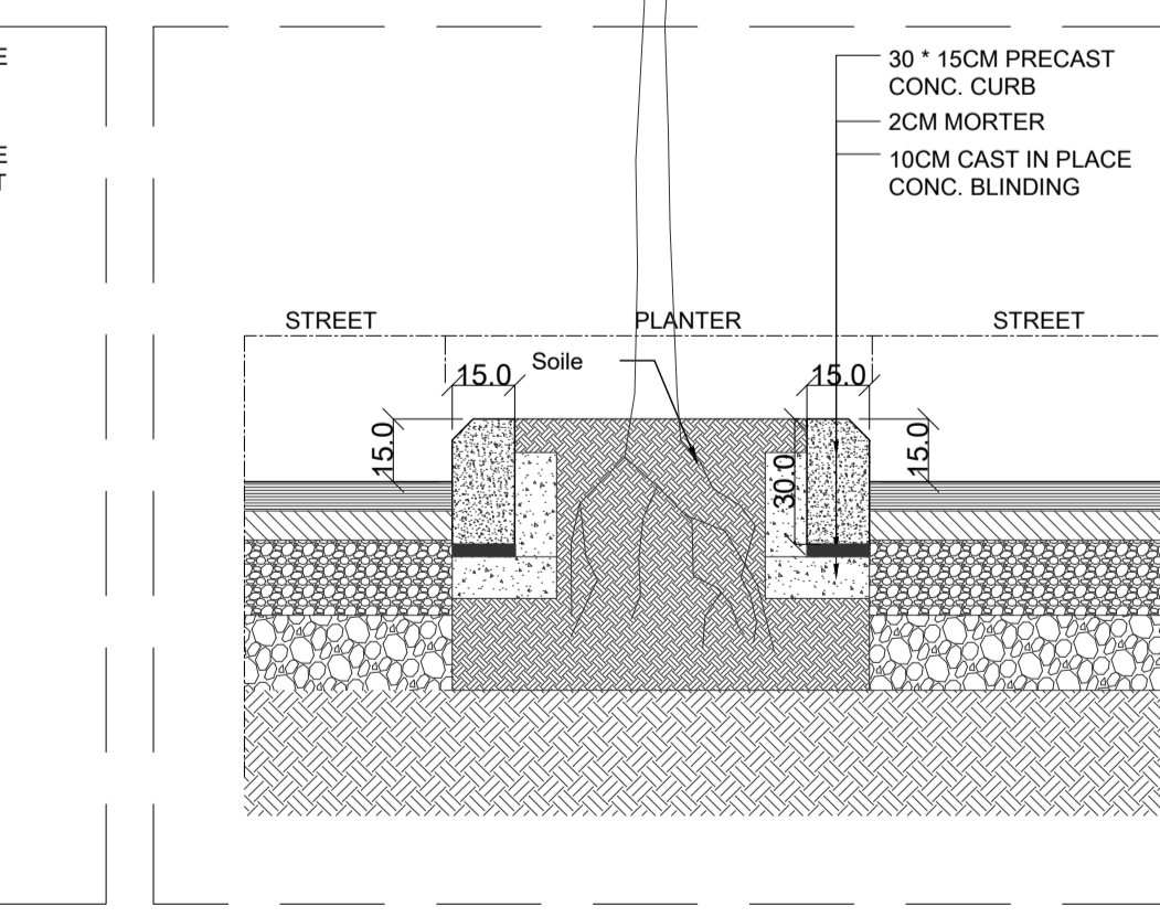
SECTION - S10 SCALE: 1-20
