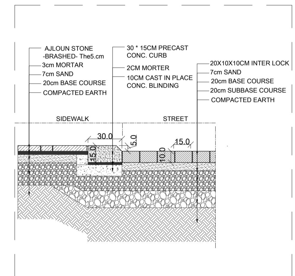
SECTION - S06 SCALE: 1-20
