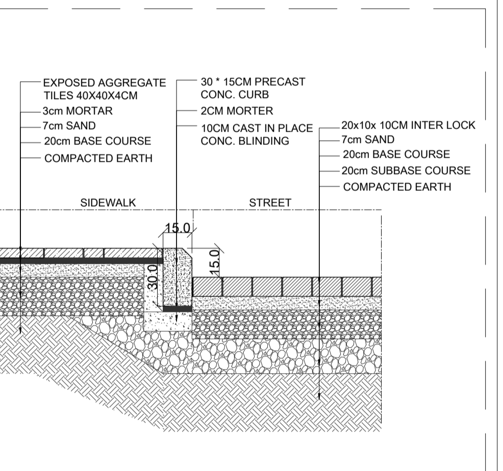
SECTION - S07 SCALE: 1-20
