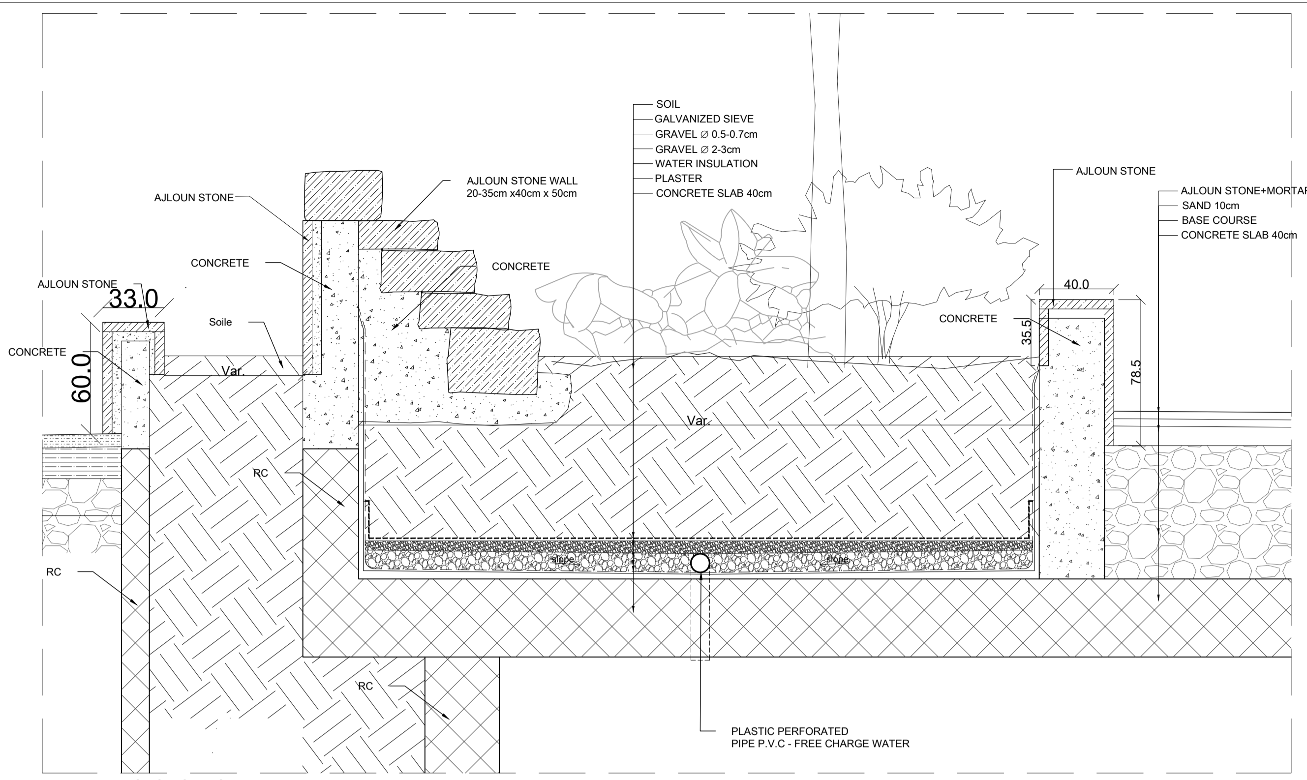
SECTION - S01 SCALE: 1/20
