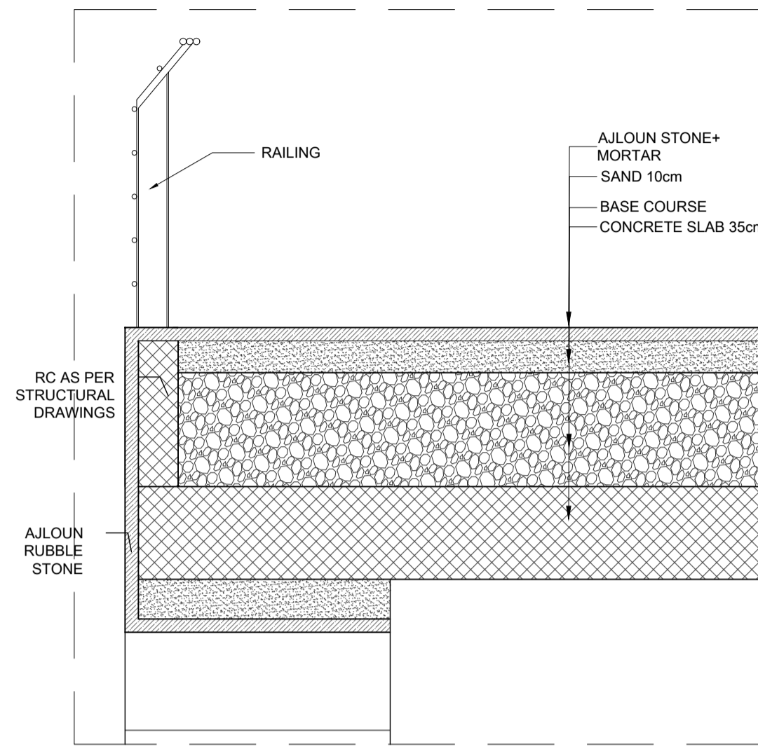
SECTION - S02 SCALE: 1-20
