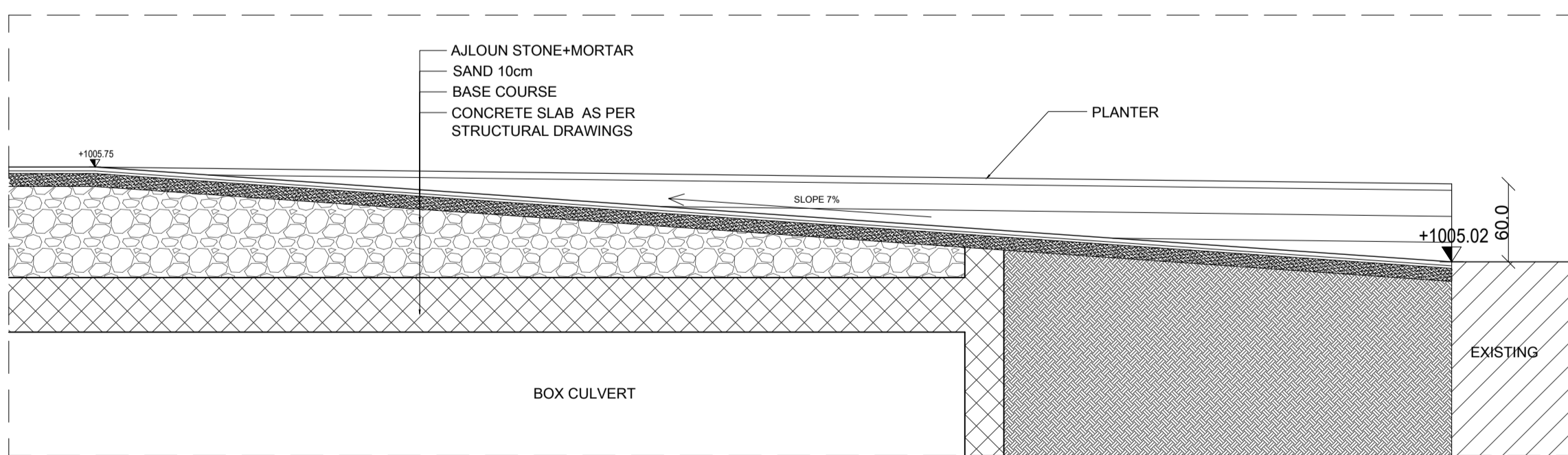
SECTION - S-18 SCALE:1-50
