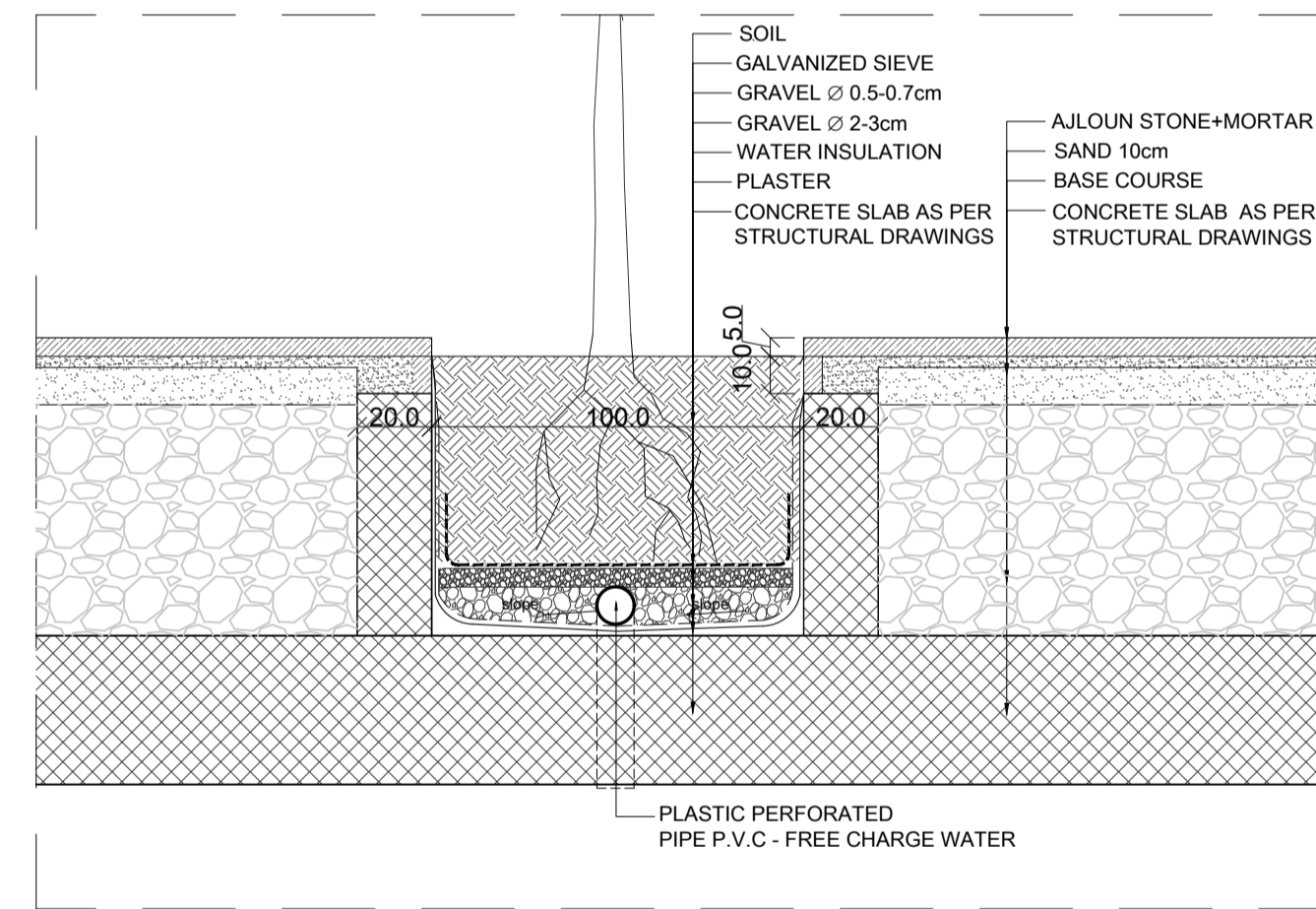
SECTION - S05 SCALE: 1-20
