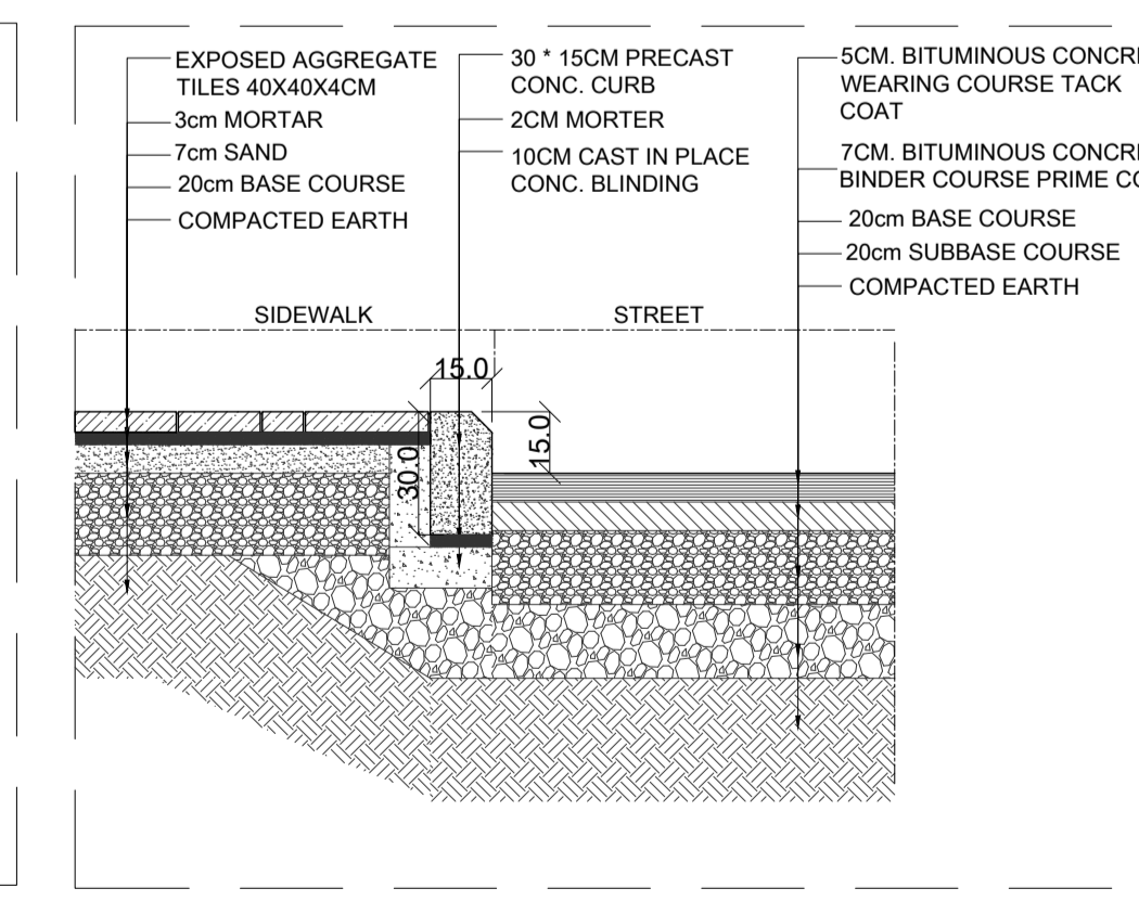
SECTION - S09 SCALE: 1-20
