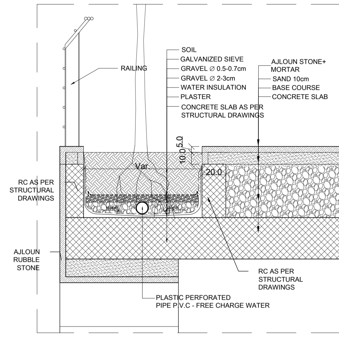
SECTION - S03 SCALE: 1-20
