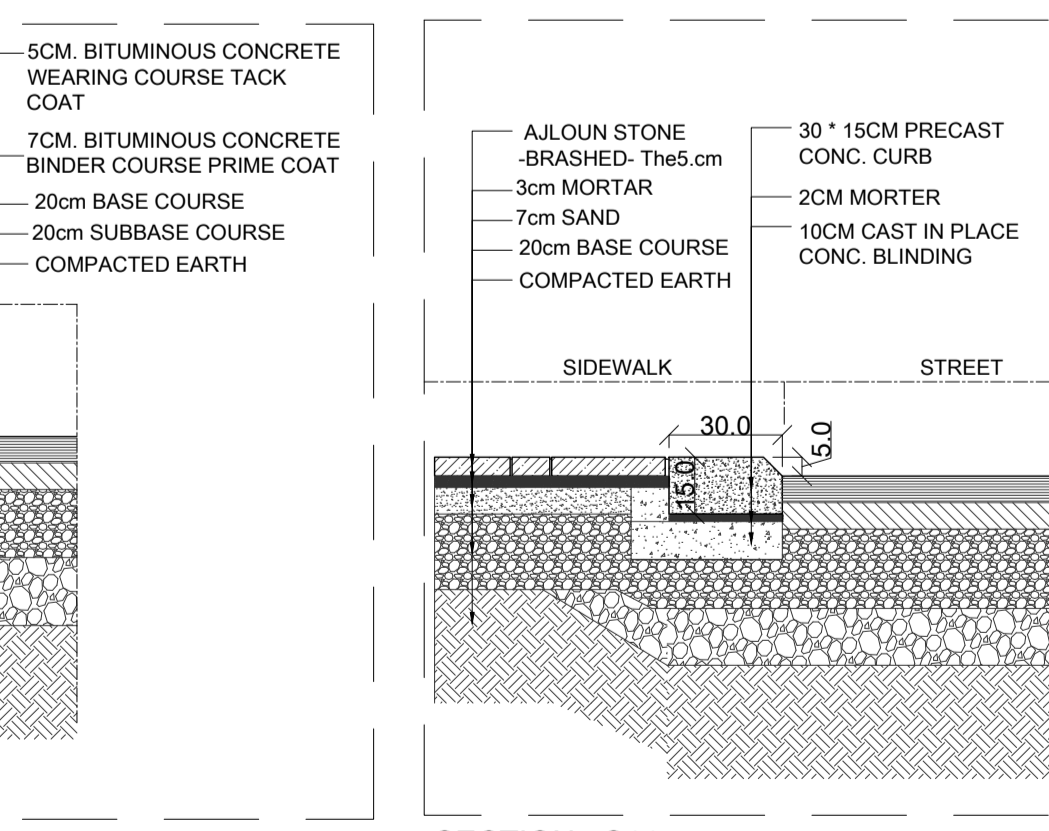
SECTION - S11 SCALE: 1-20
