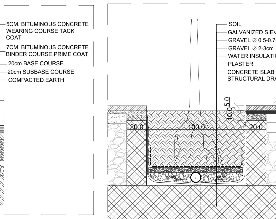
SECTION - S24 SCALE: 1-20
